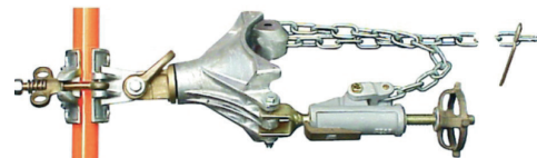
Silleta para pértiga soporte con morseto de 39 mm y extensión
