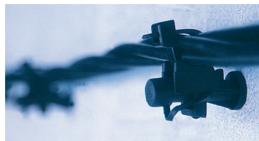
DPS25 Instalación con conductor de acometida
